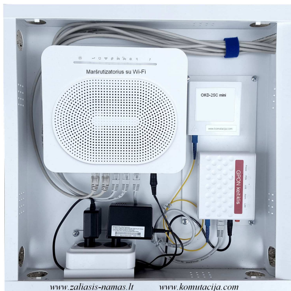
Pav.2. Galinio abonentų ryšių mazgo dėžė RMD-1 su įranga.
