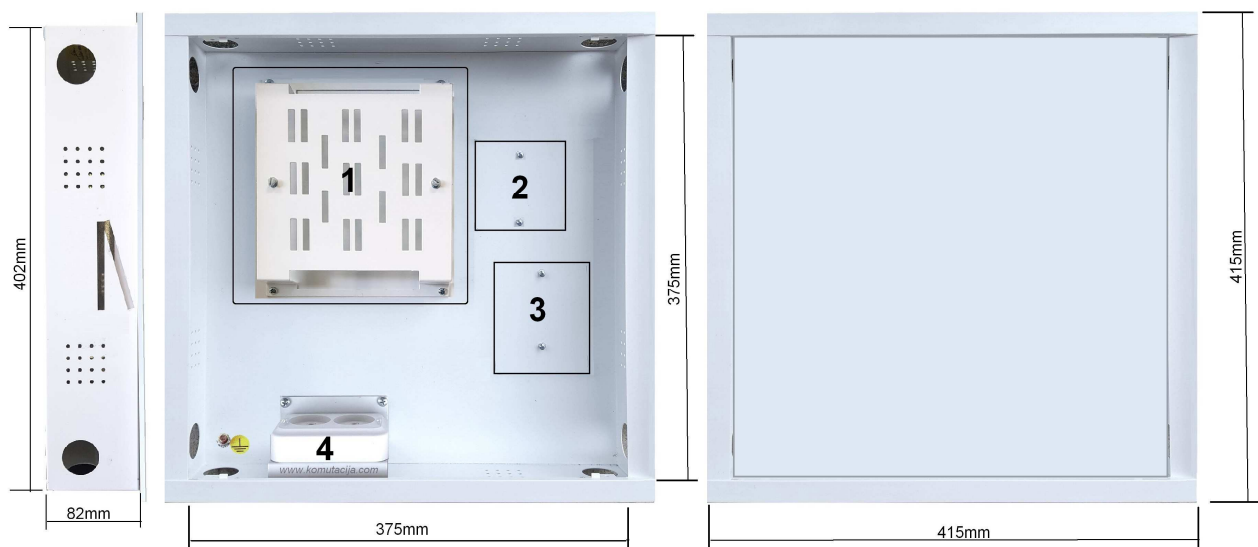
PAV.1. Galinio abonentų ryšių mazgo dėžės RMD-1 brėžinys
